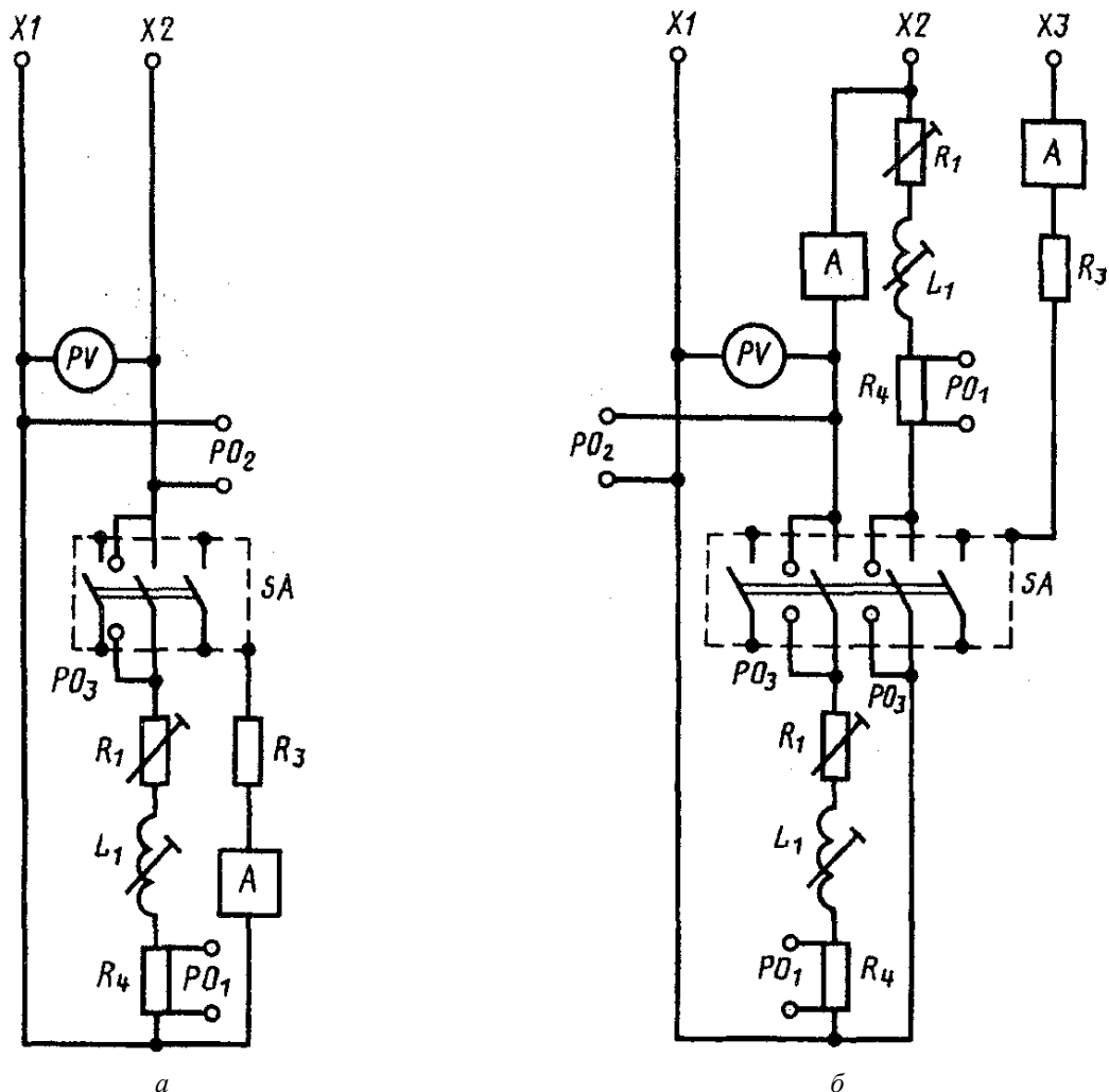
X1, X2, X3 — клеммы источника питания; PV — вольтметр; R_1 — регулируемый резистор; L_1 — регулируемые катушки индуктивности; R_3 — резистор для ограничения тока в устройстве A ; A — устройство для обнаружения перекрытий дуги; SA — испытуемый аппарат; PO_1 — осциллограф для записи тока; PO_2, PO_3 — осциллографы для записи напряжения; R_4 — шунт
