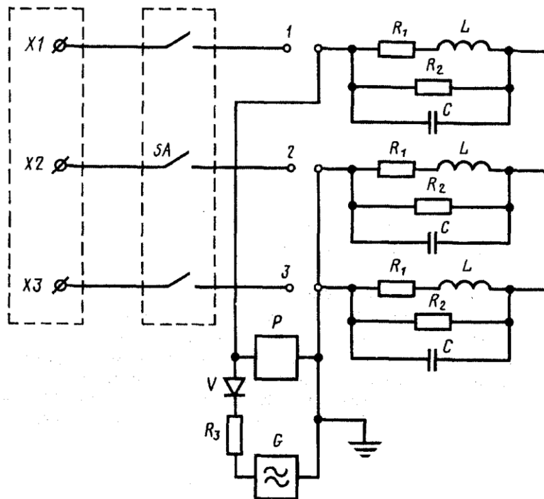
X1, X2, X3 — клеммы источника питания; SA — испытуемый аппарат; R_1 и L — активное и индуктивное сопротивление нагрузки; R_2 — шунтирующий резистор; C — шунтирующий конденсатор; P — электронный осциллограф; V — диод; R_3 — добавочный резистор; G — генератор
