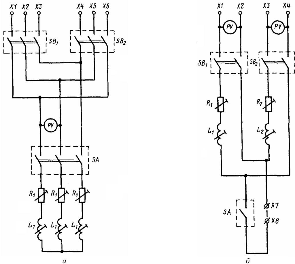
X1, X2, X3, X4, X5, X6 — клеммы источников питания; R 1 , R 2 — регулируемые резисторы; L 1 , L 2 — регулируемые катушки индуктивности; SA — испытуемый аппарат; SB 1 и SB 2 — вспомогательные аппараты; X7 и X8 — клеммы для подключения второго полюса при двухполюсном аппарате; PV — вольтметр
