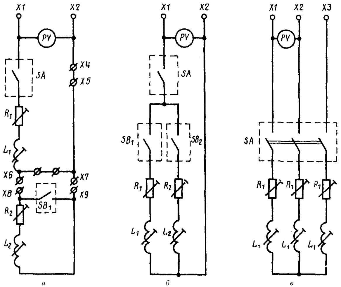
X1, X2, X3 — клеммы источника питания; R_1, R_2 — регулируемые резисторы; L_1, L_2 — регулируемые катушки индуктивности; SA — испытуемый аппарат; SB_1, SB_2 — вспомогательные аппараты; PV — вольтметр; X4, X5 — клеммы для подключения второго полюса при двухполюсном аппарате; X6, X7, X8, X9 — клеммы для подключения нагрузки при испытании в режиме АС-11 (перемычка X6-X7 должна быть снята)
