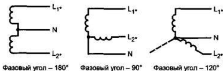
Рисунок 2 - Однофазная трехпроводная система
