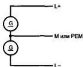
Рисунок 7 - Трехпроводная система
